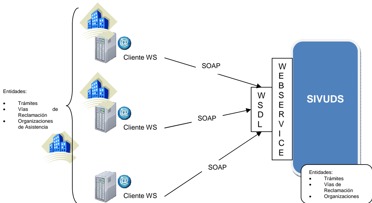
Ilustración 3 Intercambio de información mediante Web Services
