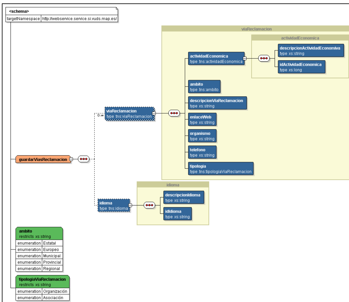
Ilustración 5 XSD Vías de Reclamación
