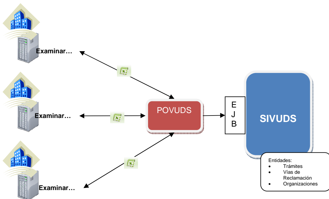
Ilustración 8 Intercambio de información mediante Ficheros
