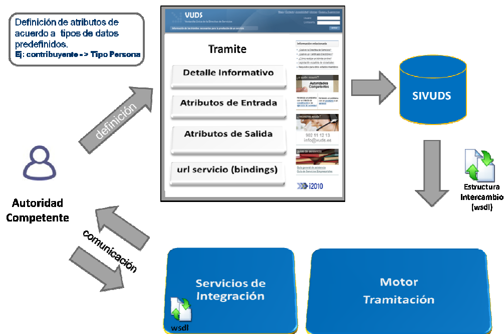
Ilustración 7 Proceso de Integración de los trámites por las AACC
