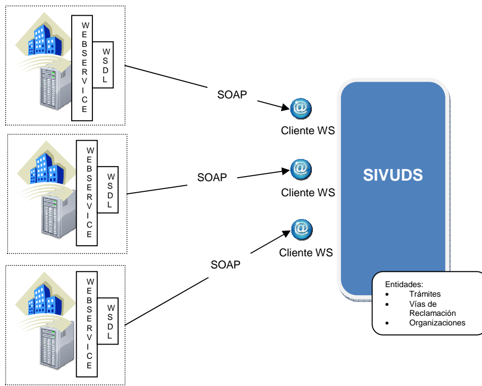
Ilustración 7 Intercambio de información mediante Web Services con AACC sin servicios para intercambio
