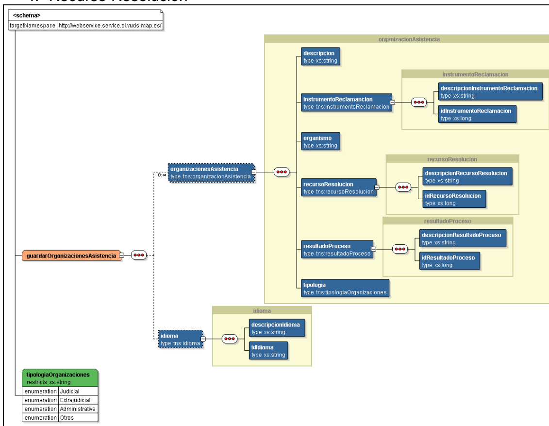
Ilustración 6 XSD Organizaciones de Asistencia
